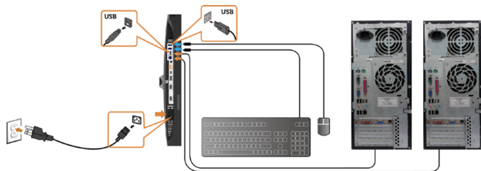
b. 2つのコンピュータの接続
